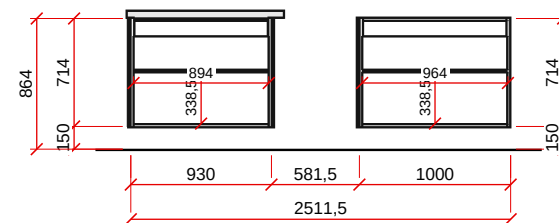
VISTA D - ESC. 1:50
