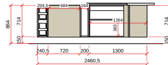
VISTA B - ESC. 1:50
